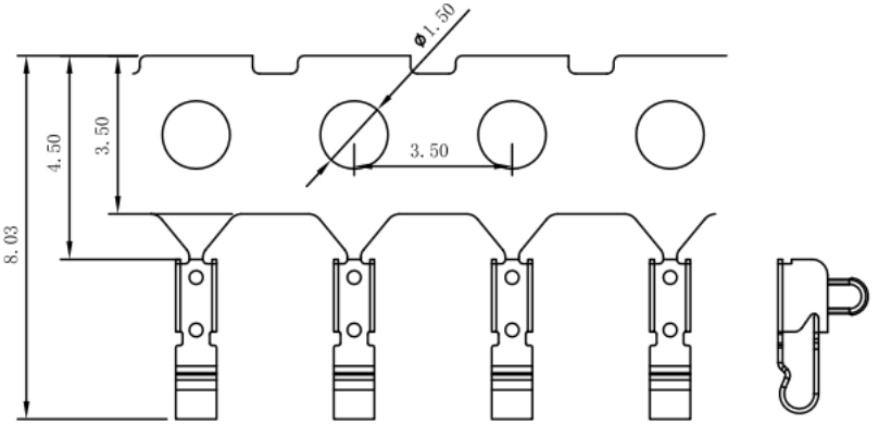
料带示意图 比例: 1/2
