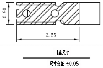
料带示意图 比例: 1/2
