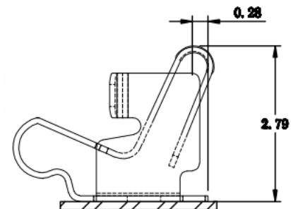
极限工作高度 B=2.8 \text{ mm}
