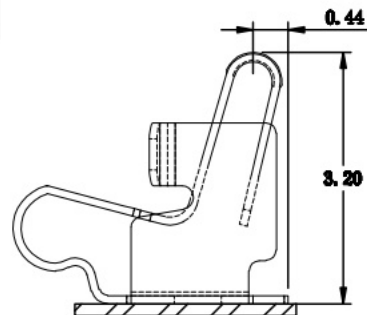
正常工作高度 B=3.20
