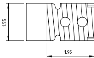
焊盘位置 尺寸公差 ±0.05
