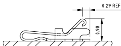
正常工作高度 H=0.90
