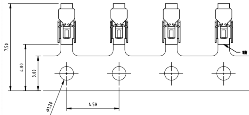
料带示意图 比例: 1/2
