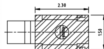
焊盘尺寸 尺寸公差 ±0.05
